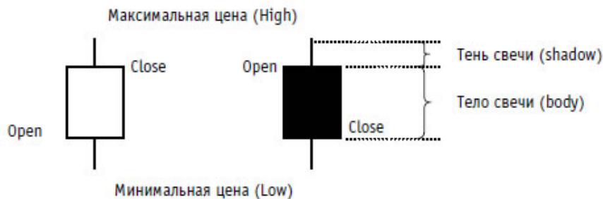
Рис. 2.6. Схематичное отображение японских свечей
