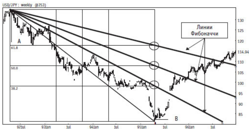
Рис. 2.90. Веерные линии Фибоначчи на чарте USDJPY с 1992 по 1996 г.
