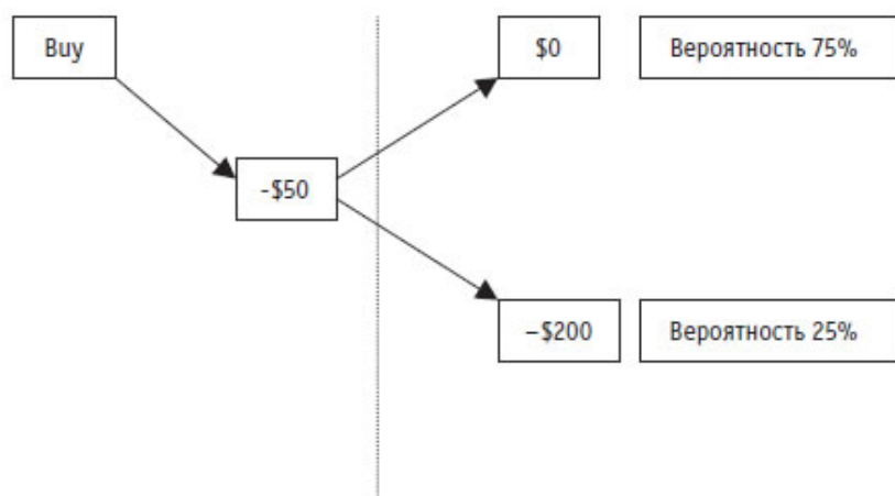
Рис. 4.5. Схематичное соотношение вероятности и финансового результата
