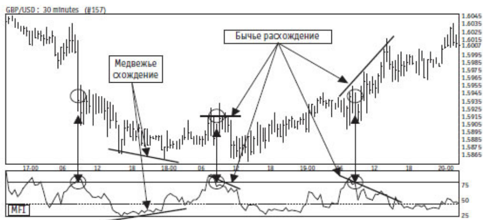
Рис. 2.71. Пример анализа MFI
