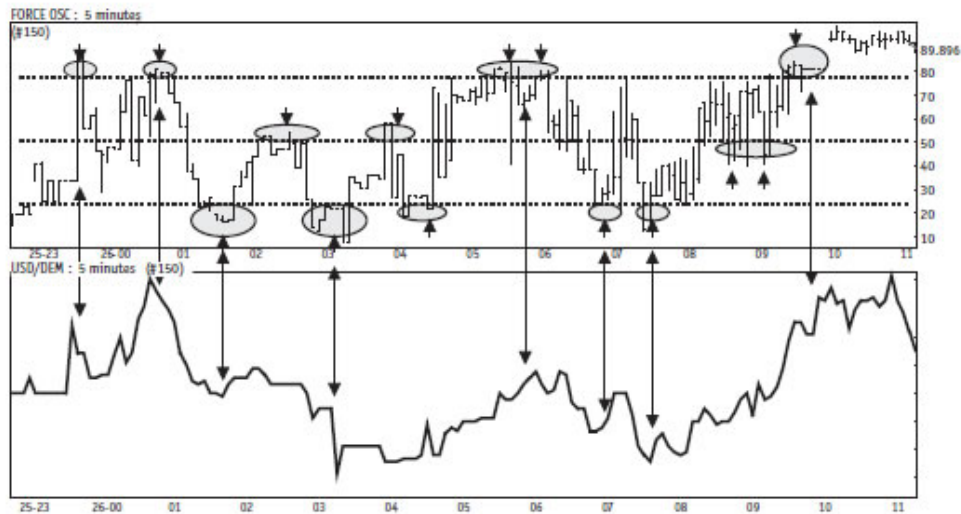
Рис. 2.146. Сила осциллятора
