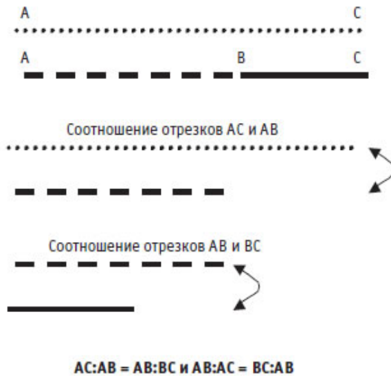
Рис. 2.89. Золотое сечение
