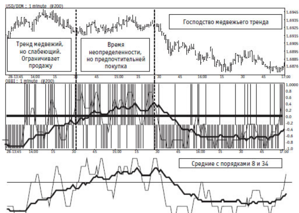
Рис. 2.122. Анализ индикатора OBVI
