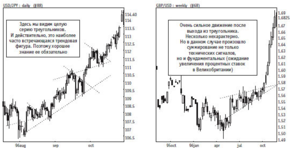
Рис. 2.28. Примеры фигуры «сходящийся треугольник»
